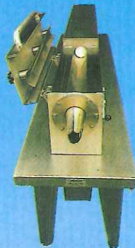
EMBUCHADORAS SEMI-AUTOMÁTICAS DE LOMOS CURADOS Y COCIDOS EPM-200
