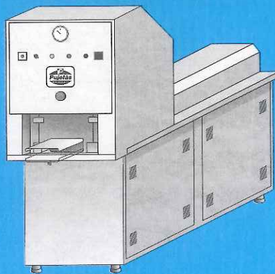
PRENSA FORMADORA DE JAMONES CURADOS DESHUESADOS (SISTEMA RECTANGULAR PARA LONCHEAR CON MERMA 0) PF-4000
