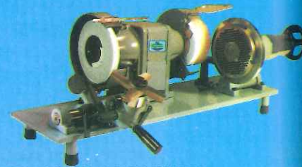
RECTIFICADORA PARA PLACAS Y CUCHILLAS DE PICADORA RCP-70/200
